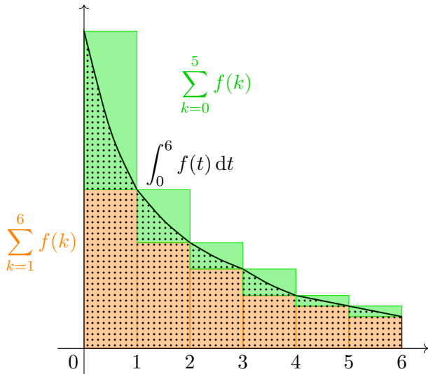
FIGURE 2 – Exemple de comparaison série-intégrale pour une fonction f décroissante, positive.
