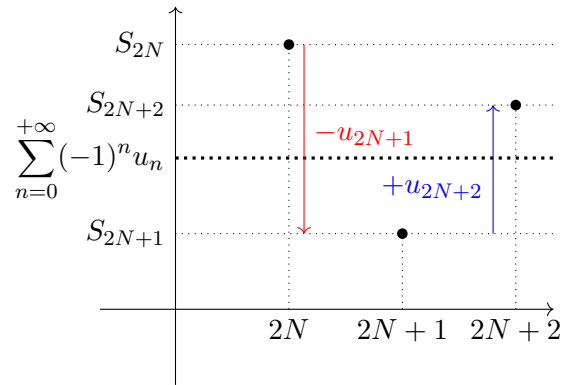
FIGURE 4 – Illustration de l'adjacence de (S_{2N})_{N \in \mathbb{N}} et de (S_{2N+1})_{N \in \mathbb{N}} .
