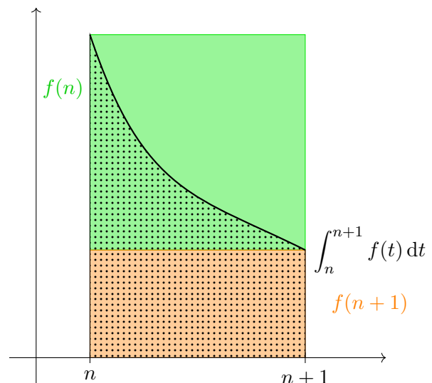
FIGURE 1 – Comparaison série-intégrale pour encadrer l'intégrale, sur un intervalle [n, n+1] .
